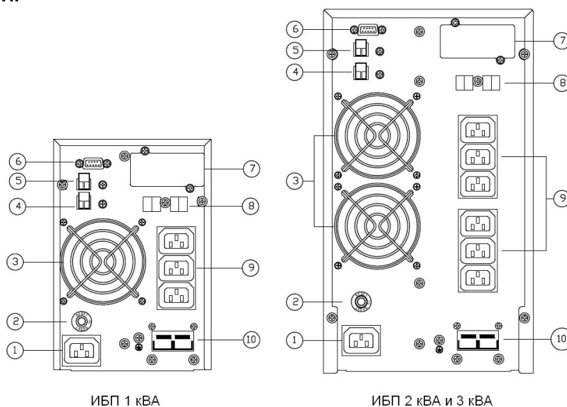
ИБП 1 кВА
